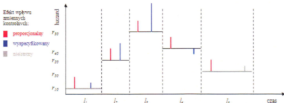
Wykres 1. Rodzaje efektów zmiennych kontrolnych w modelu wykładniczym przedziałami stałym
