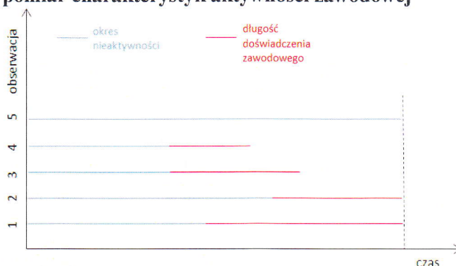
Wykres 2. Definicja i pomiar charakterystyk aktywności zawodowej
